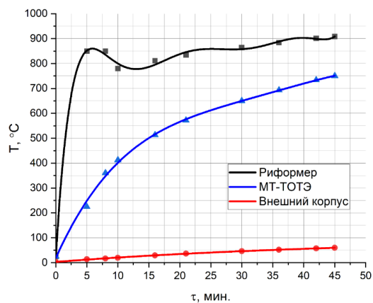
Рисунок 1 - График выхода узлов ЭХГ на рабочие температуры. Расход топлива (пропан-бутановой смеси) – 300 мл/мин. На 5-ой минуте работы риформера в режиме полного окисления, был снижен поток воздуха до \lambda=0.7 .
