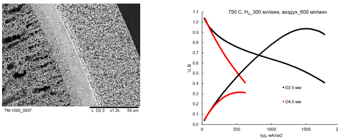
Рисунок 1 – Микроструктура МТ ТОТЭ и его вольтамперные характеристики.
